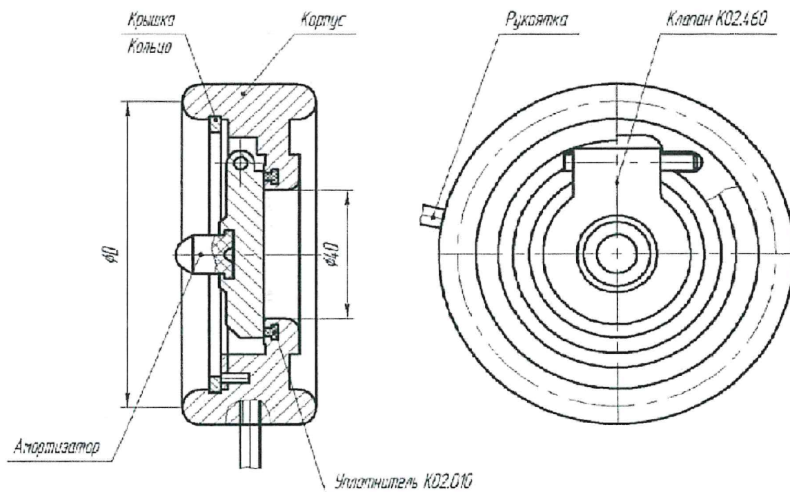
Рисунок 1 – Клапан обратный
